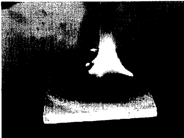
Fotografie dell'accensione della provetta secondo la norma NF P92-501.
